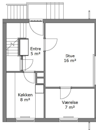
Stueplan, eksisterende 1 : 100
