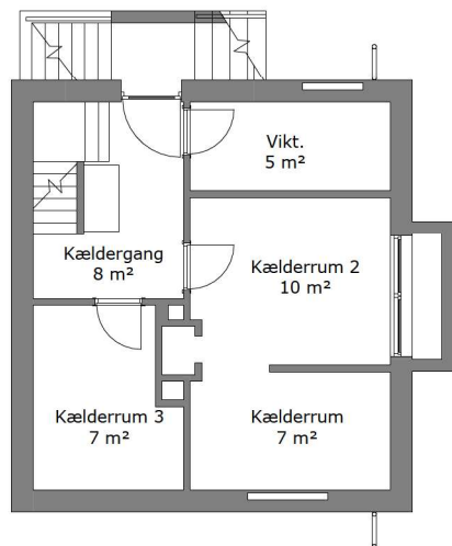
Kælderplan, eksisterende 1 : 100
