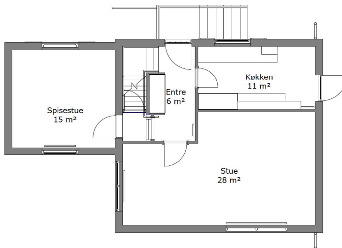
Stueplan, eksisterende forhold 1 : 100
