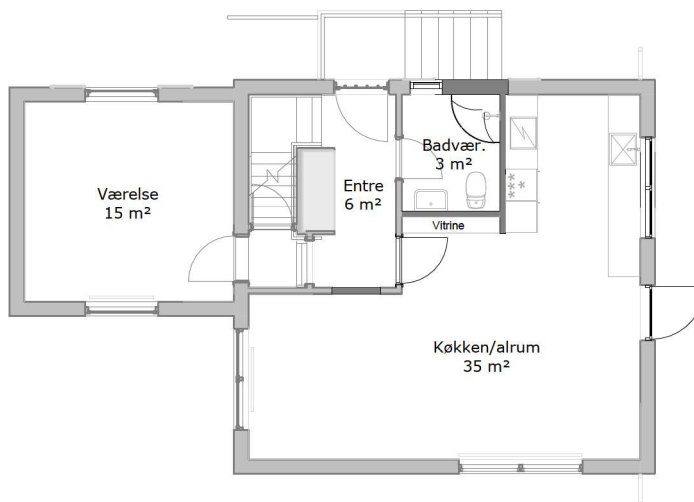
Stueplan, , ny forhold 1 : 100
