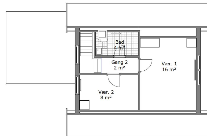
1.sal, eksisterende forhold 1 : 100
