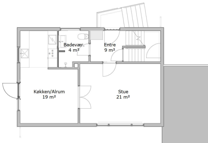
Stueplan, nye forhold 1 : 100
