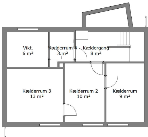
Kælderplan, eksisterende 1 : 100
