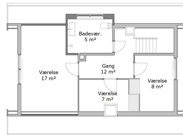
1.sal, nye forhold 1 : 100
