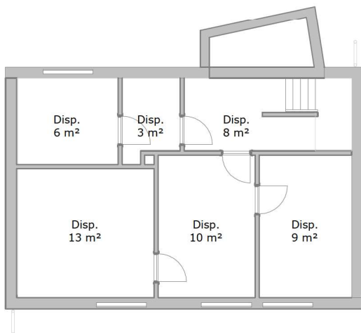
Kælderplan, nye forhold 1 : 100
