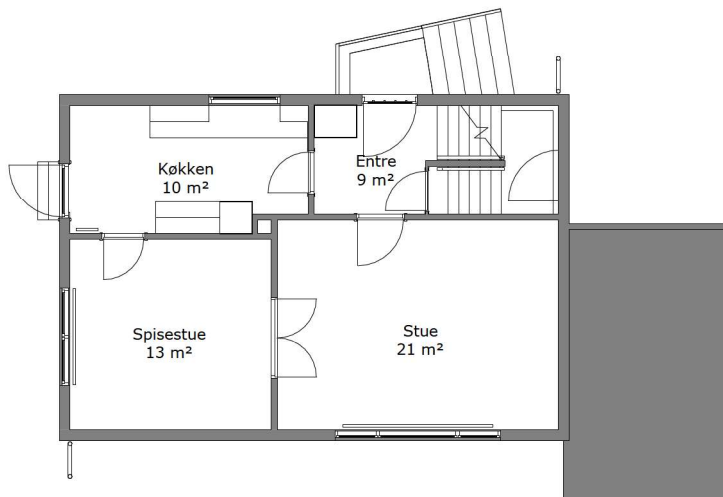
Stueplan, eksisterende 1 : 100
