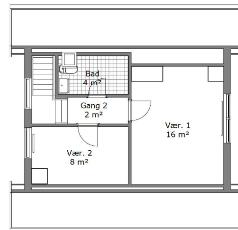
1.sal, eksisterende 1 : 100
