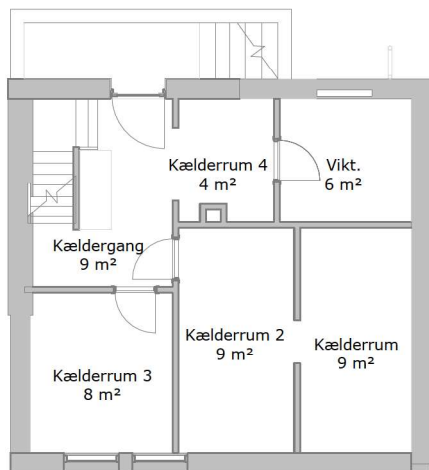
Kælderplan, nye forhold 1 : 100
