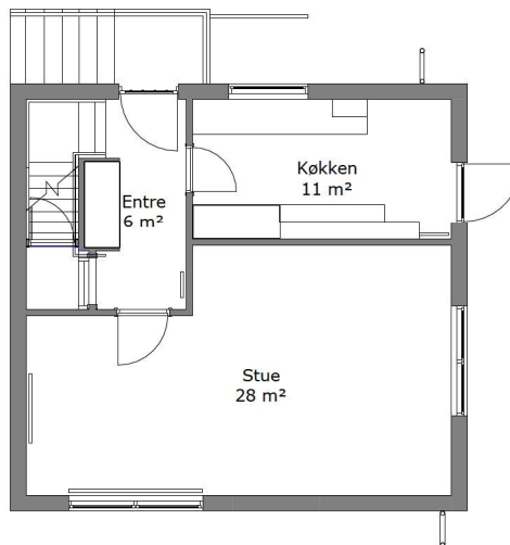
Stueplan, eksisterende 1 : 100
