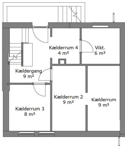
Kælderplan, eksisterende 1 : 100
