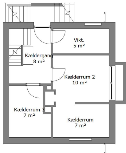
Kælderplan, eksisterende forhold 1 : 100
