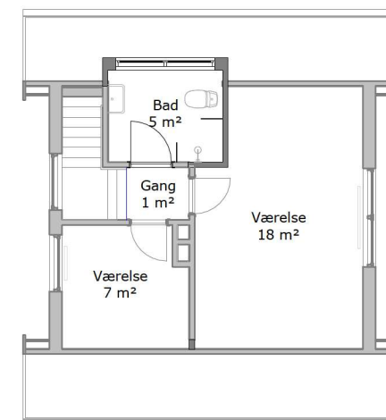
1.sal, nye forhold 1 : 100
