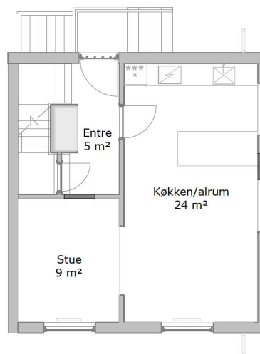
Stueplan, nye forhold 1 : 100
