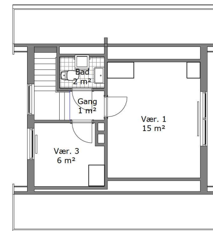
1.sal, eksisterende forhold 1 : 100
