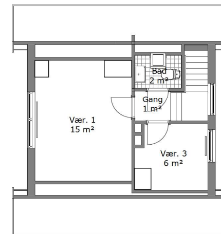
1.sal, eksisterende forhold 1 : 100
